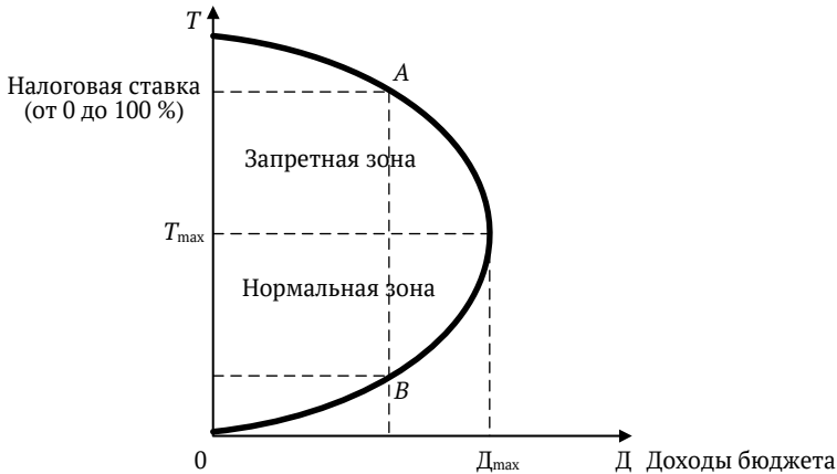
Рис. 1. Кривая Лаффера:
